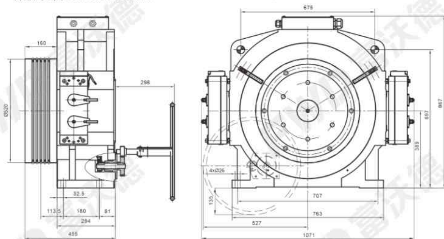
外形尺寸图 Overall Dimensions
