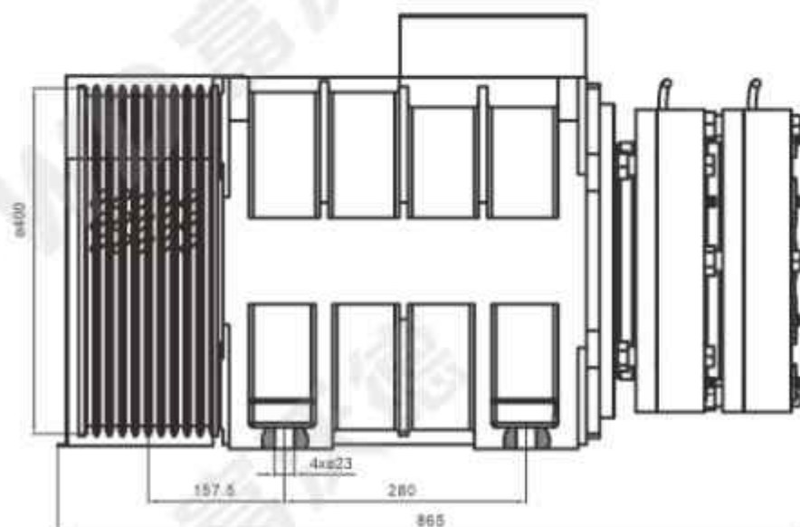
外形尺寸图 Overall Dimensions
