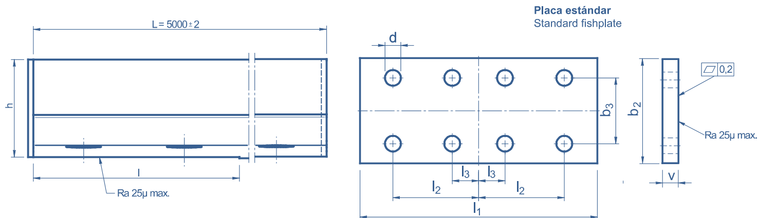
Placa estándar Standard fishplate Placas especiales en catálogo Placas de Unión. Special fishplates in Fishplates catalogue.
