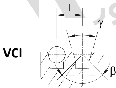
gole a V con sottointaglio V grooves with undercut
