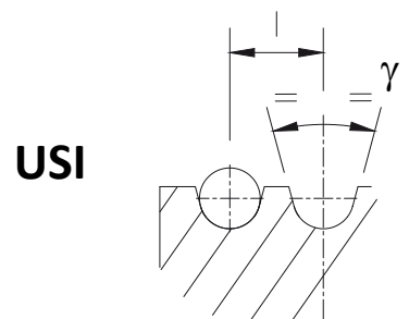
gole a U senza sottointaglio U grooves without undercut
