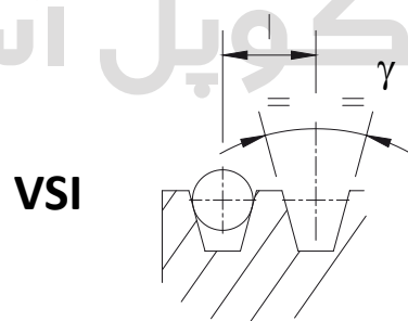
gole a V senza sottointaglio V grooves without undercut
