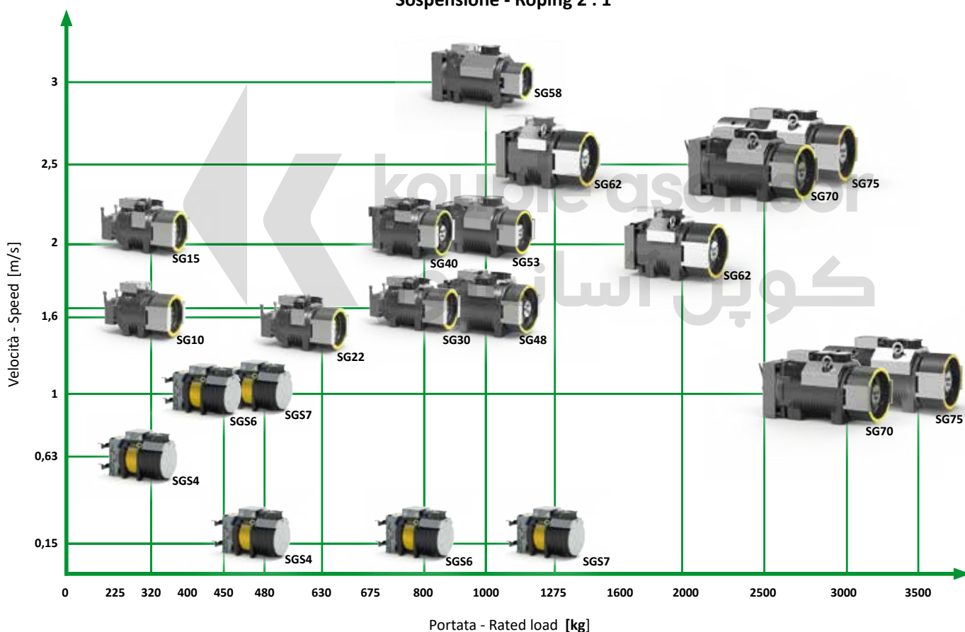
Sospensione - Roping 2 : 1
