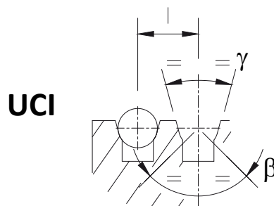
gole a U con sottointaglio U grooves with undercut
